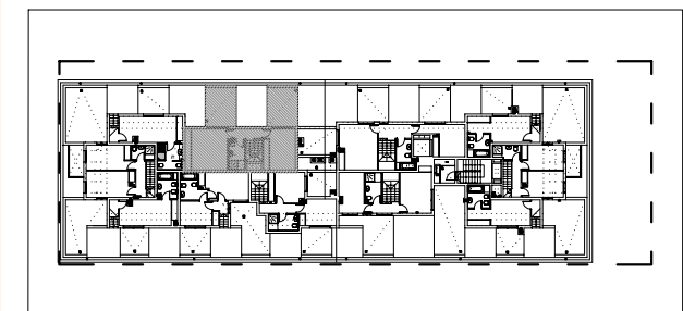
PLANTA BAJOCUBIERTA
